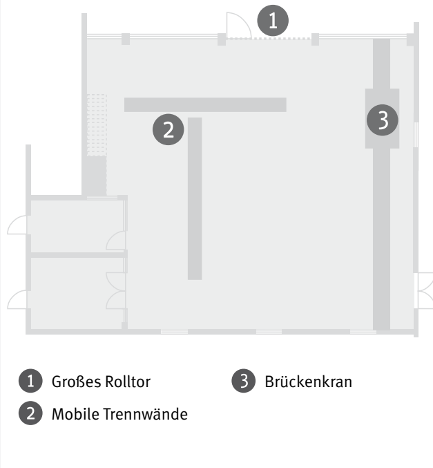
Grundriss der Mehrzweckhalle
