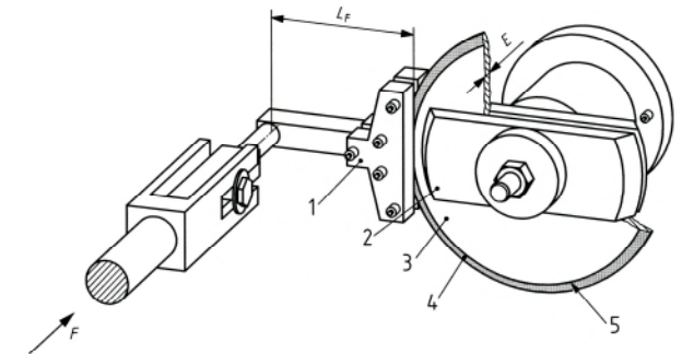
Legende 1 Klemmstück 2 Spannplatte 3 Grundkörper 4 Segment 5 Verbindungszone
