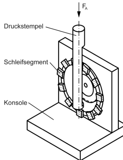
Prüfvorrichtung zur Ermittlung der Abscherkraft
