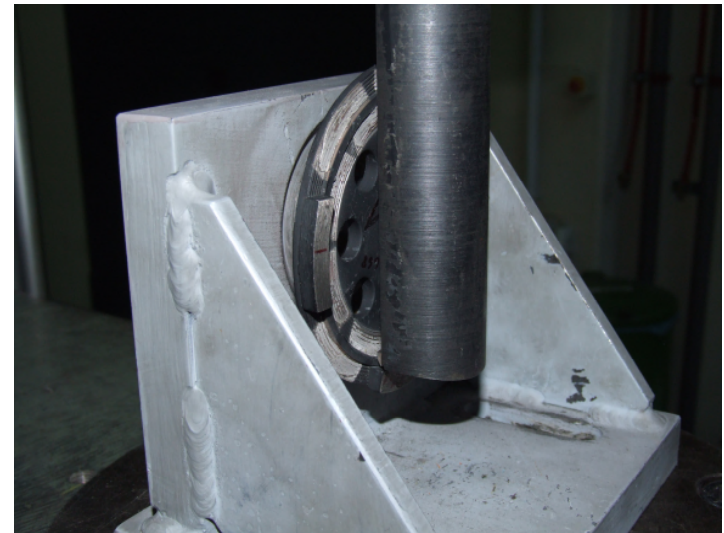
Prüfvorrichtung zur Ermittlung der Abscherkraft
