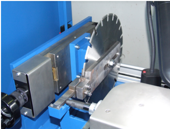
Biegeprüfmaschine für segmentierte und geschlossene Diamant-Trennscheifscheiben
