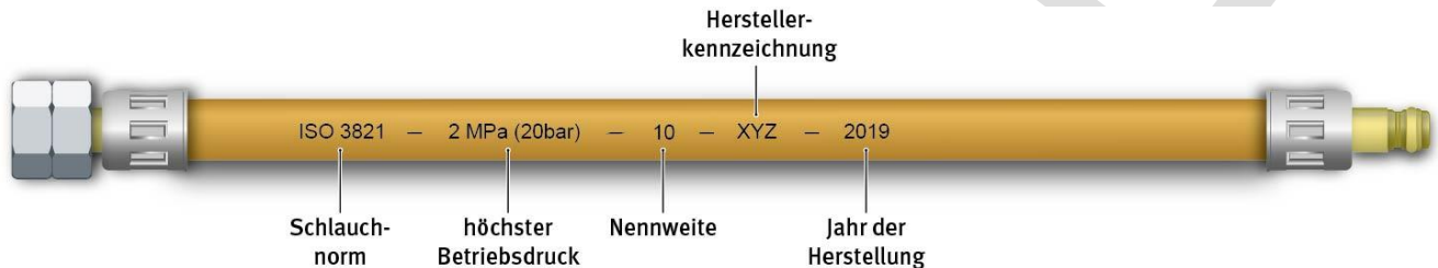
Bild 9: Kennzeichnung von Schlauchleitungen
