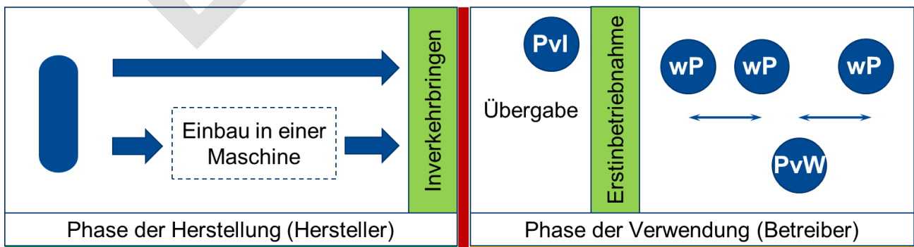
Abbildung 2 – Lebensphasen eines Hydrospeichers (Abkürzungen siehe Begriffe, Seite 5)
