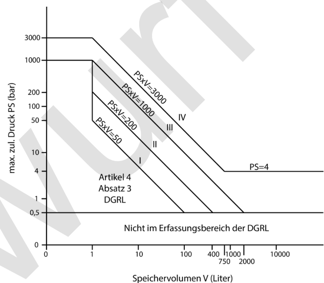
Abbildung 4 – Diagramm 2 nach Anhang II der DGRL für Behälter für Gase (auch überhitzte Flüssigkeiten) der Fluidgruppe 2
