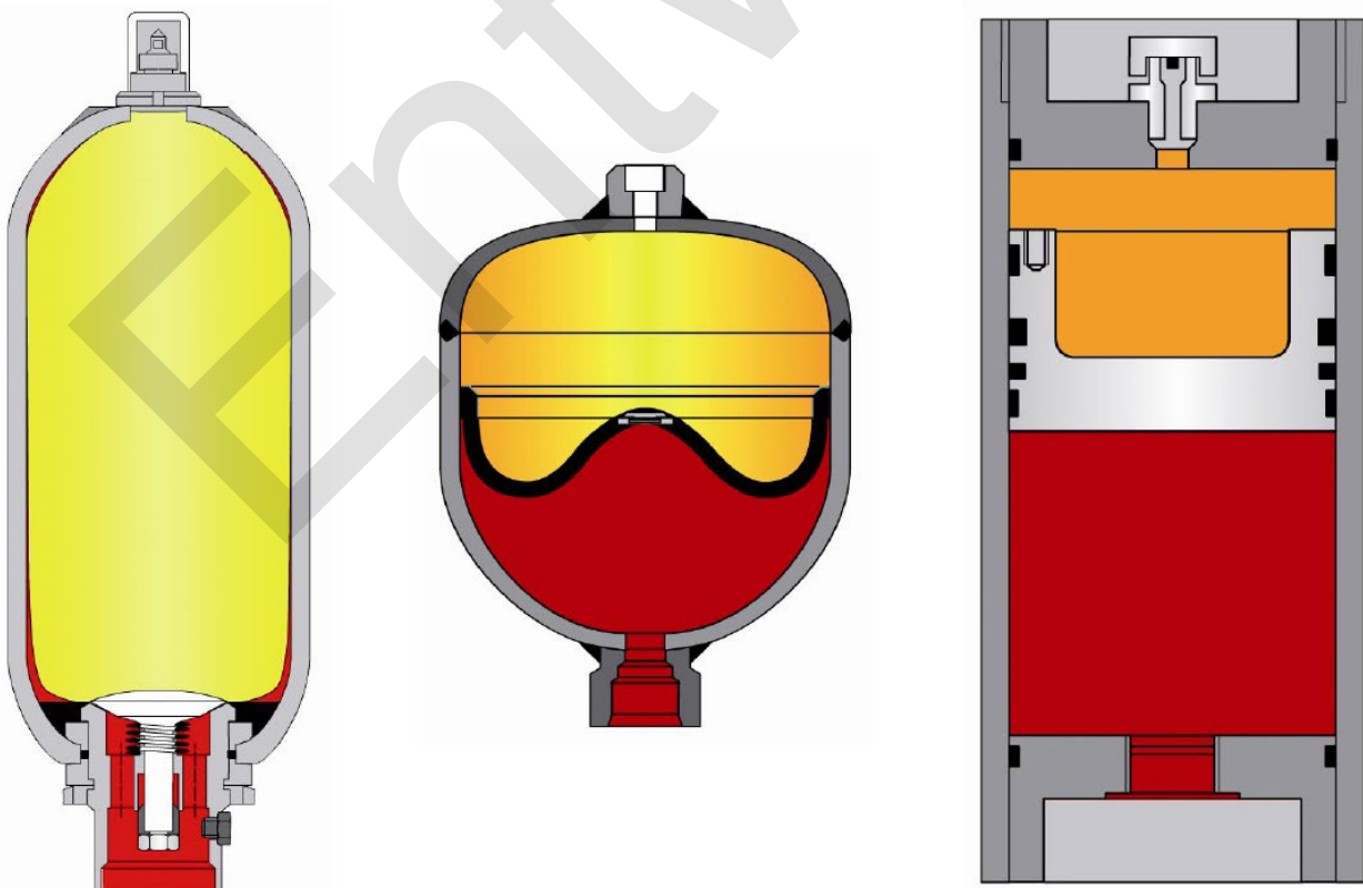
Abbildung 3 – Blasenspeicher leer (Links), Membranspeicher gefüllt (Mitte), Kolbenspeicher gefüllt (Rechts)
