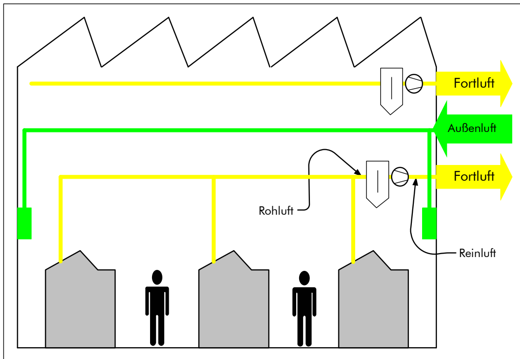
Abbildung 3: Hallenquerschnitt
